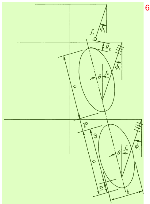
图 6 导线舞动时的电气间隙 7
