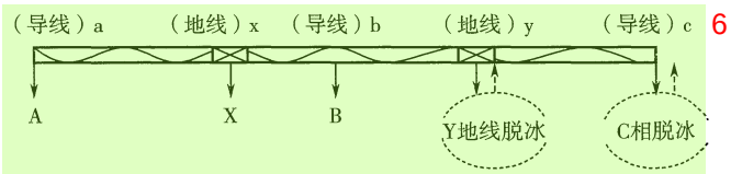
图 9 不均匀冰荷载组合示意图 7
