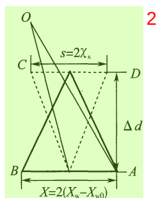
图 5 脱冰雪导线的运动范围示意图
