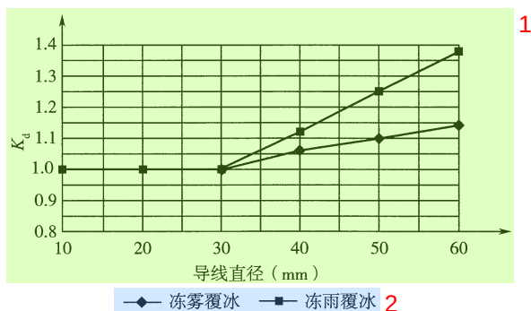
图 1 导线直径相关的系数 K_d
