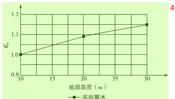
图 2 和导线高度相关的系数 K_h
